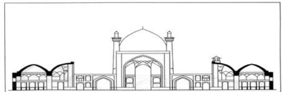
اصفهان، مسجد امامی نما - برش
