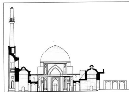
یزد، مسجد جامع، برش و نما ( ژویر ) .
