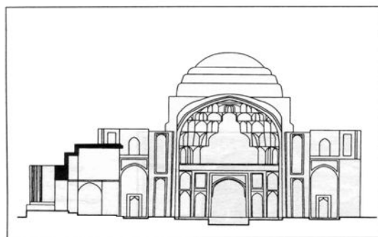
مسجد جامع ورامین، نما — برش (از مرکز لند نقشه معماری و شهرسازی دانشگاه علم و صنعت ایران).
