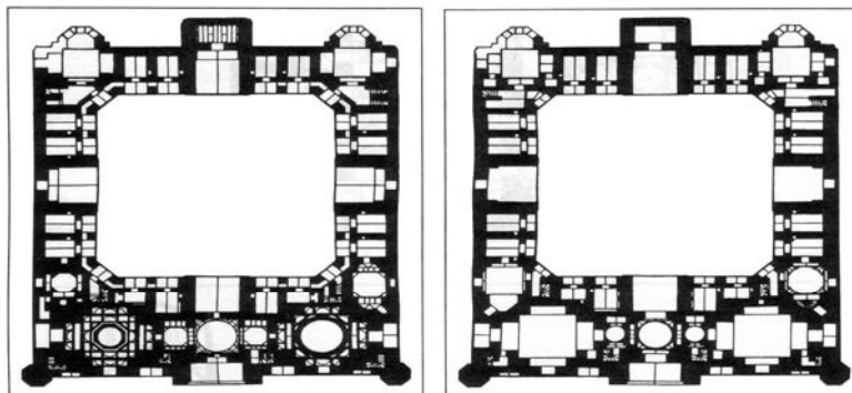
خواف، مدرسه غیاثیه خرگرد، طبقه همکف و اول، اثر معماران قوام‌الدین و غیاث‌الدین شیرازی (از معماری اسلامی دوران تیموری، همکف و ویرا).
