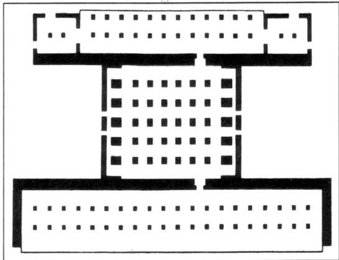
پاسارگاده نقشه کاخ اختصاصی کوروش
